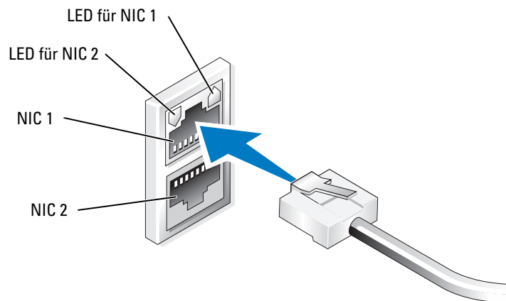
Abbildung 1-1. NIC-Anschluss
